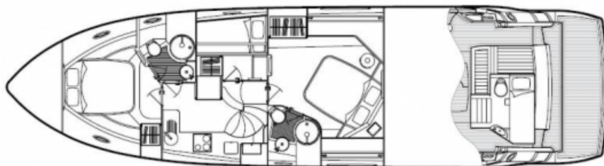
Pont inférieur
