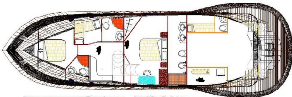
layout ponte inferiore esempio combinazione 3+1
