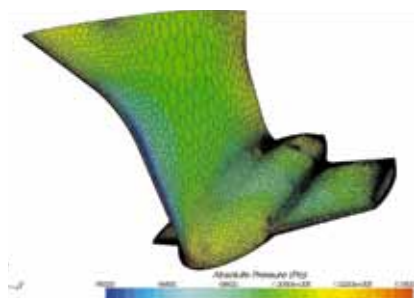
Advanced winged keel design for shoal draft version Quille optimisée, à ailettes, pour la version PTE Fortschrittliches Flügelkiel Design für Kurzkielversion Quilla corta optimizada con aletas Chiglia ottimizzata, con alette, per la versione ridotta
