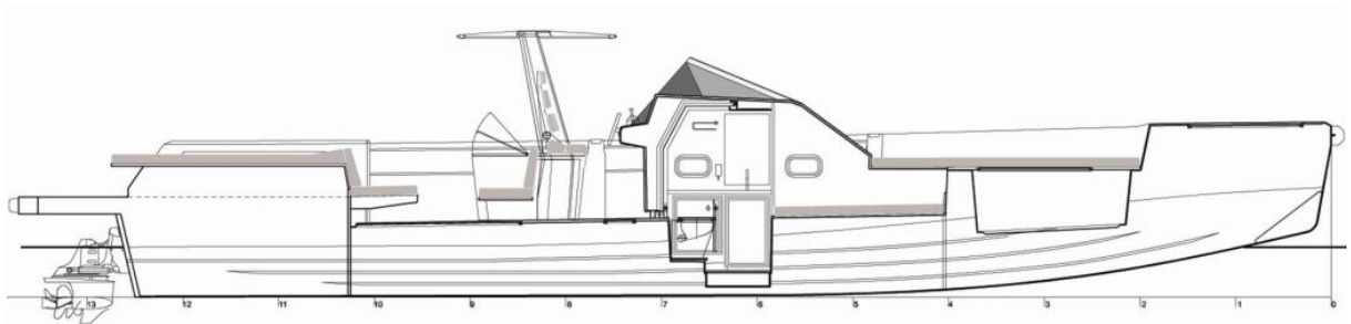
Longitudinal Section
