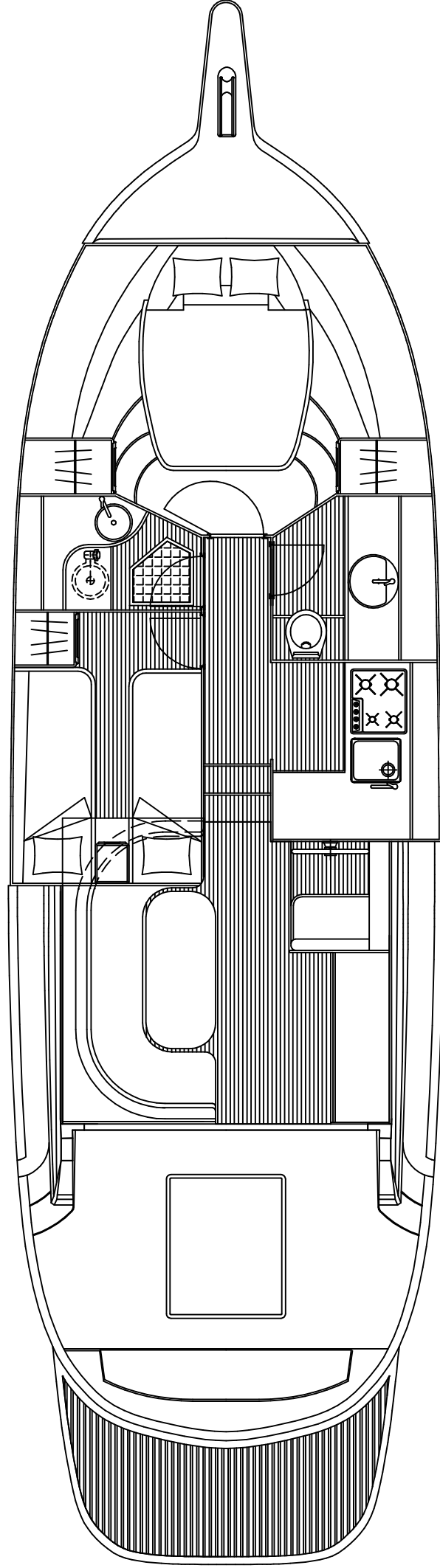
Sciallino 40 - 2 cabine
