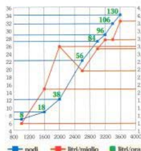
RELAZIONI TRA NUMERO DI GIRI - VELOCITÀ - CONSUMI - AUTONOMIA
