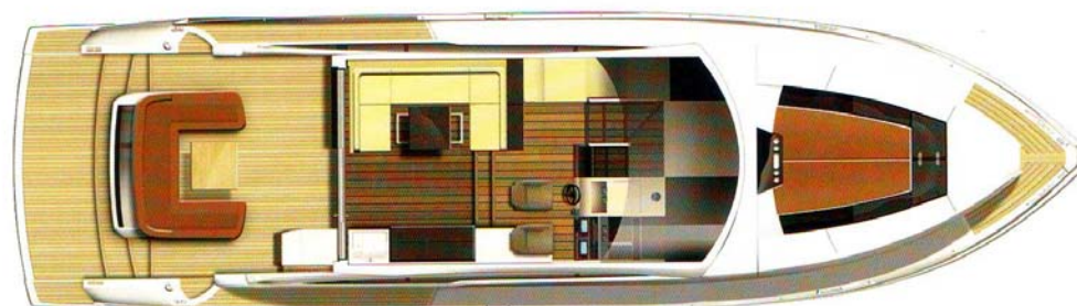
Layout del ponte, del pozzetto e del salone
