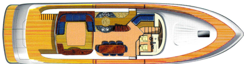
Pianta del salone opzionale con divano fisso e panche fisse nella sala da pranzo.
