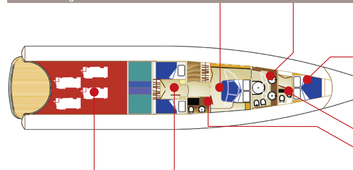
Sala macchine
