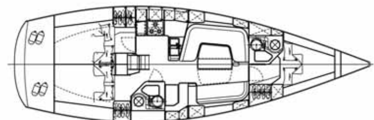
Versión 3-camarotes, segundo baño. Versione 3-cabine con due bagni.
