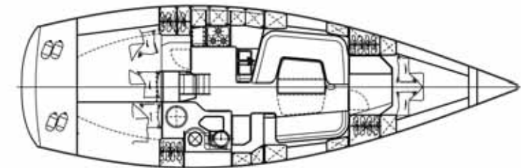
Versión 2-camarotes, camarotes a estribor en popa con colchones y espacio para almacenaje. Versione 2-cabine con cabina di poppa a tribordo con materasso e deposito.
