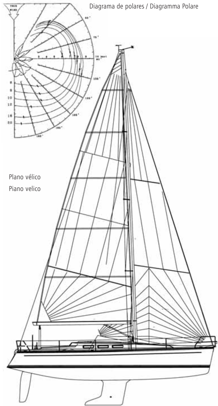
Diagrama de polares / Diagramma Polare
