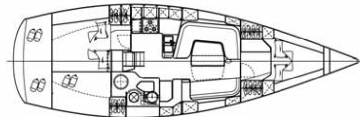
Versión estándar 2-camarotes. Versione 2-cabine standard.
