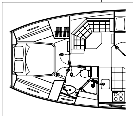
Salone inferiore opzionale in luogo della terza toilette
