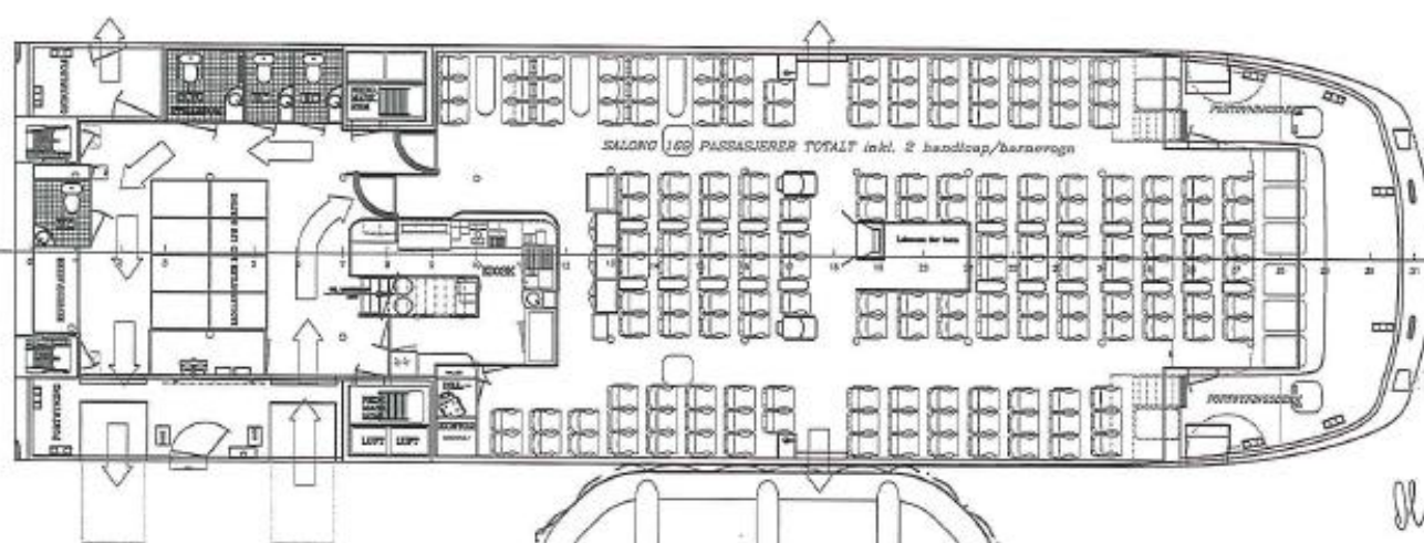
PLAN HOVEDDEKK
