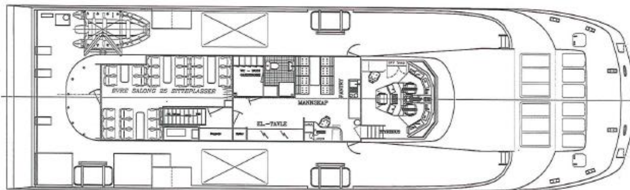
PLAN BRODEKK
