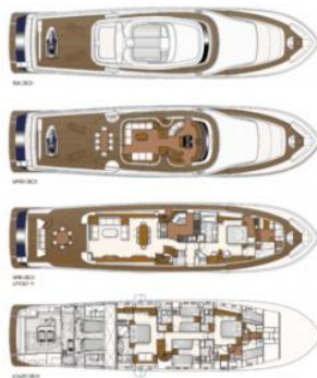
Lay-out Cabins
