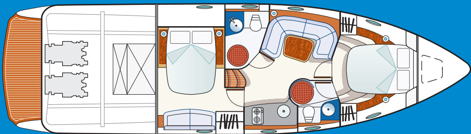
versione 2 cabine 2 cabins
