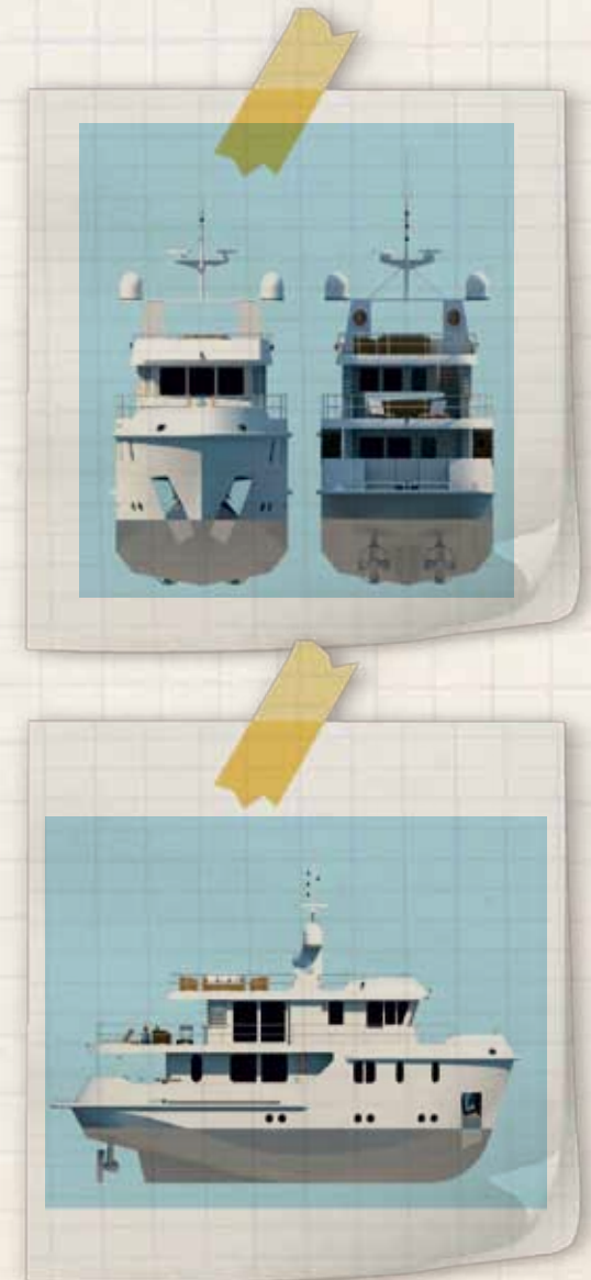
figura 1: Eliche protette dallo Skeg. Anche urtando un grosso ostacolo non si danneggerebbe l'elica.
