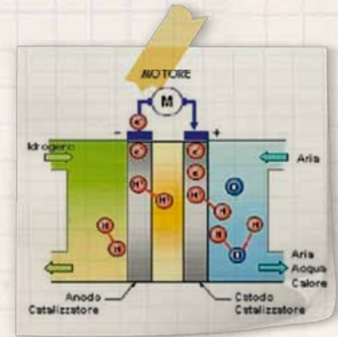
Schema di funzionamento a Fuel Cell
