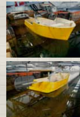
figura 2: Modello Ocean King in Vasca Navale
