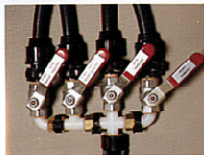
Les vannes à quart de tour montées sur tuyauterie rigide.
