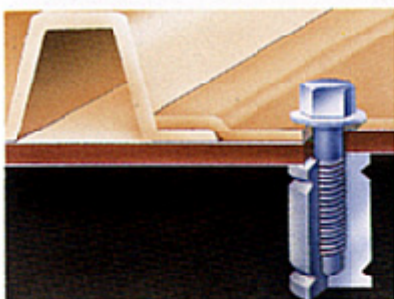
Fixation du lest avec insert en acier.
